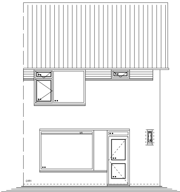
VOORGEVEL
